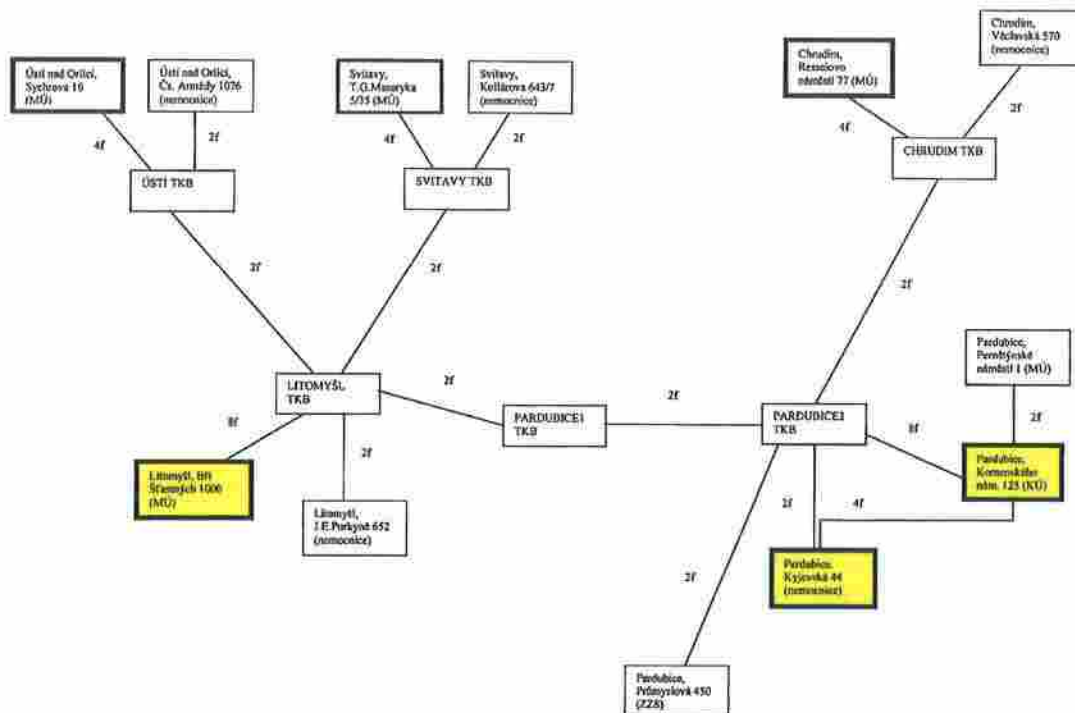
Obrázek 1 – Fyzická topologie RDS – přehled vláken
