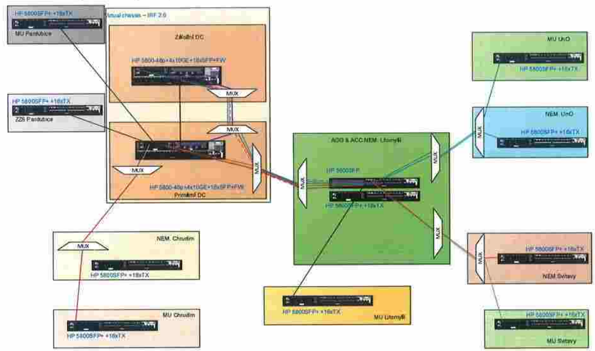
Obrázek 2 – Fyzická topologie RDS
