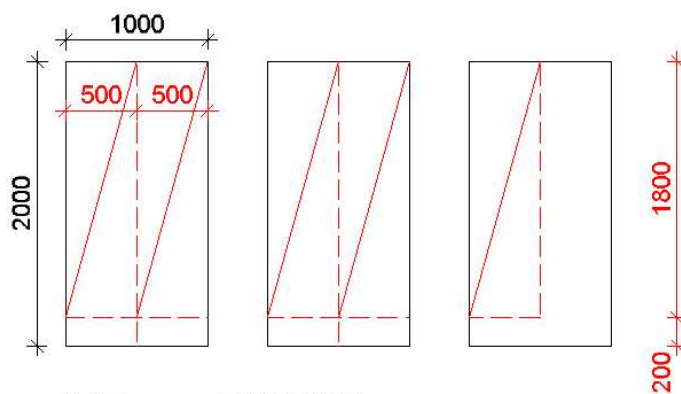
3 plechy nerezové 1,5/1000/2000
