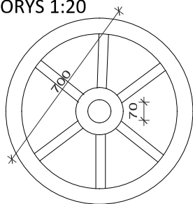
PŮDORYS 1:20
