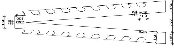
ŘEZ 1:20
