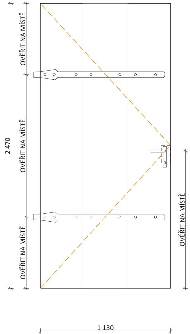
VNITŘNÍ POHLED M 1:20
