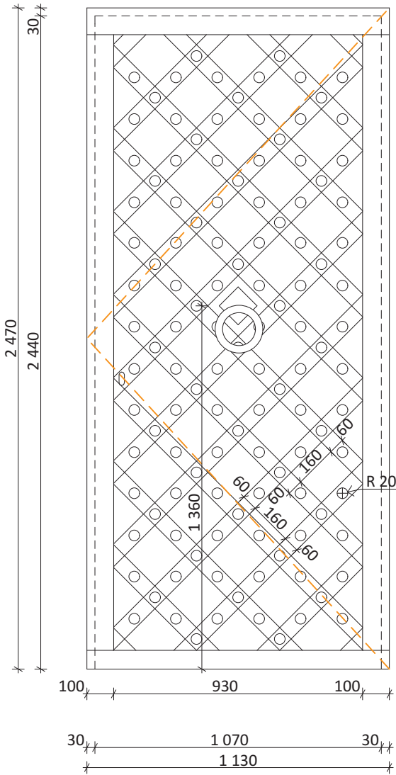
ČELNÍ POHLED M 1:20
