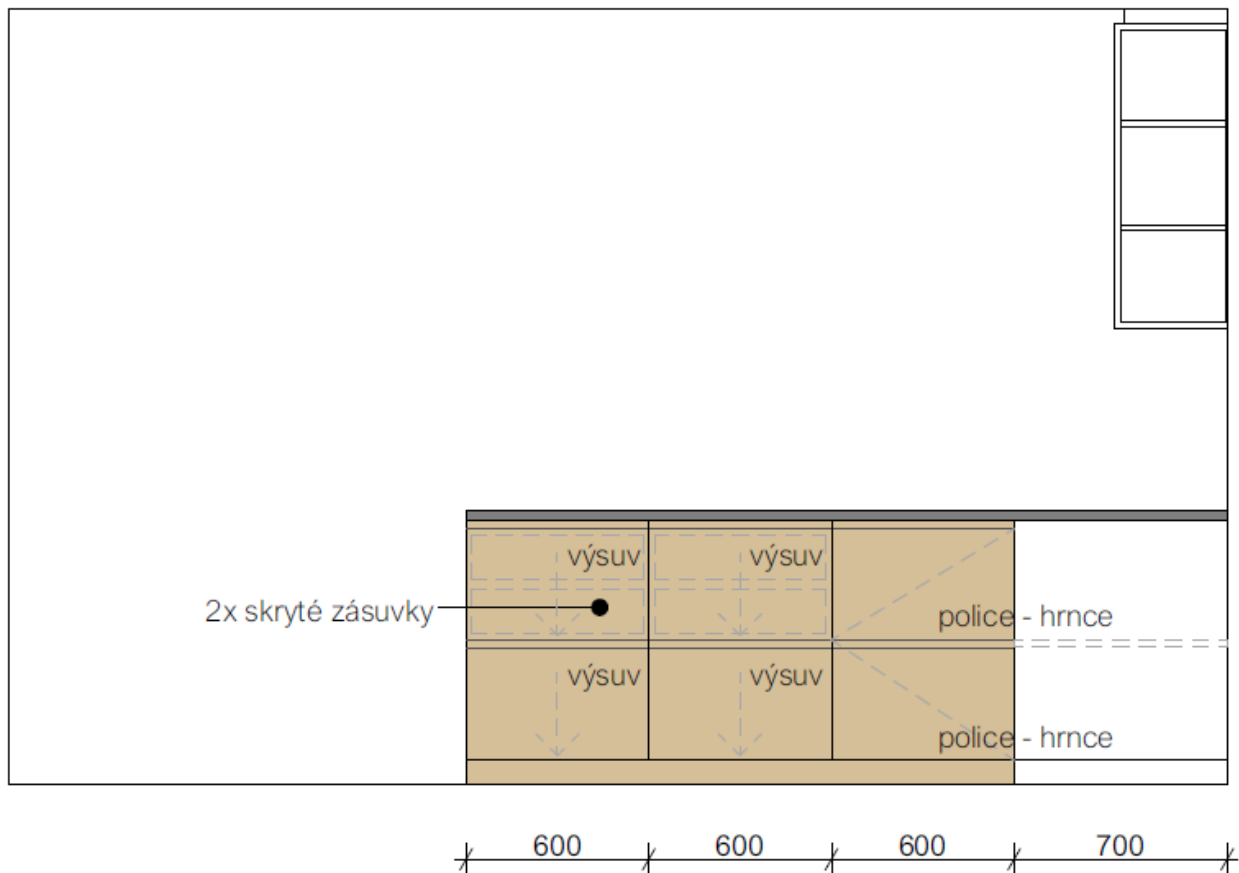
pohled K3
