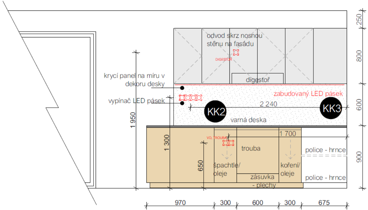
pohled K2
