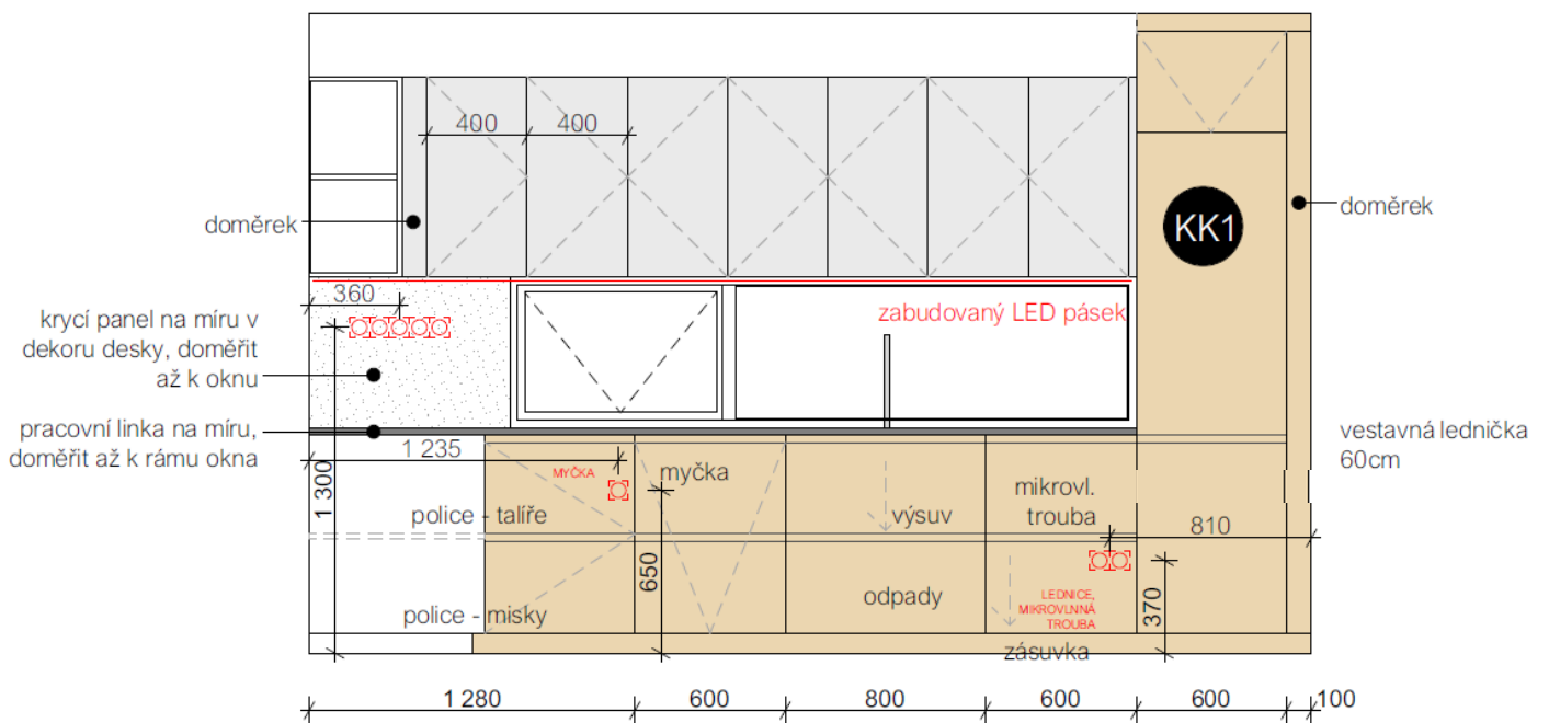
pohled K1
