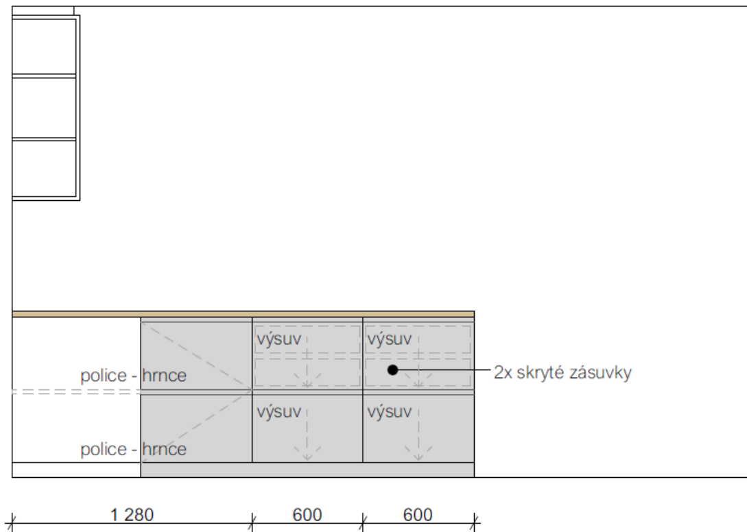
pohled K3
