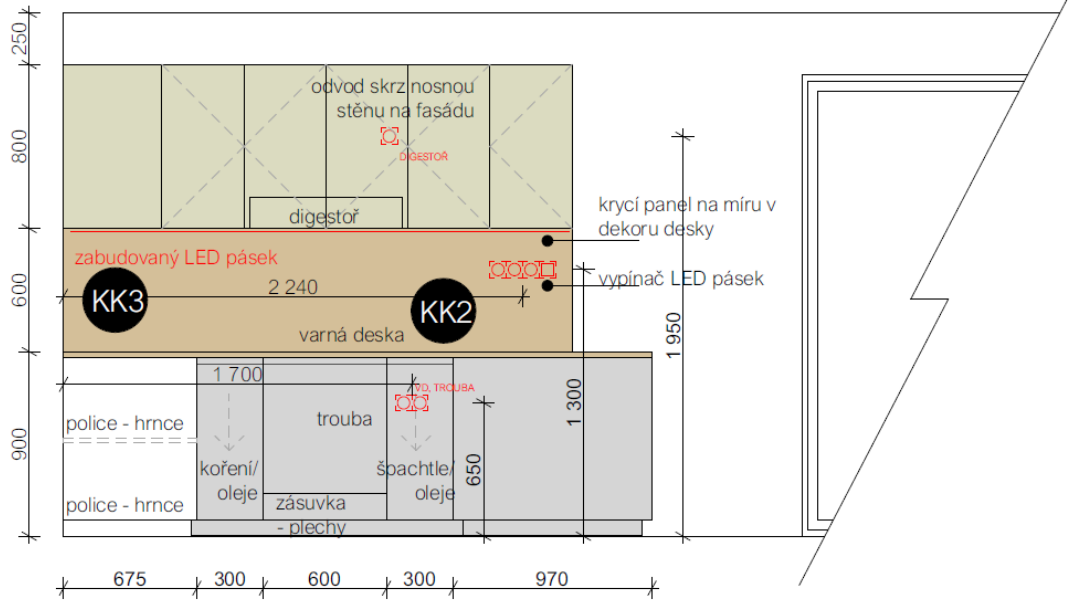
pohled K2
