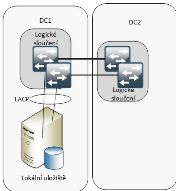
Obrázek 2 – minimální způsob zapojení v DC1
