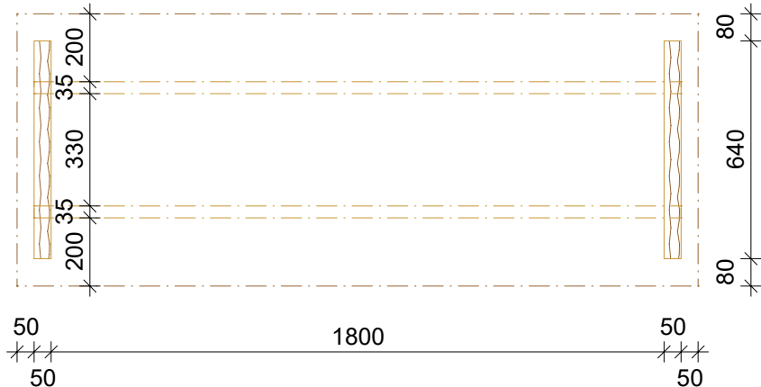
PŮDORYS
