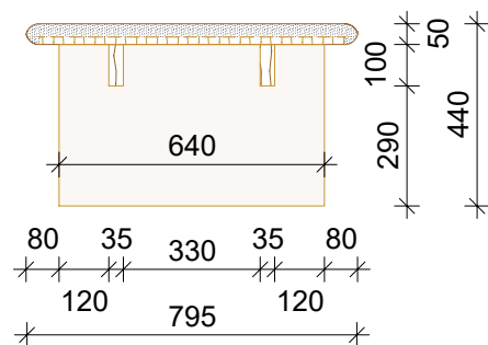
POHLED C
