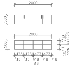
PŮDORYS
