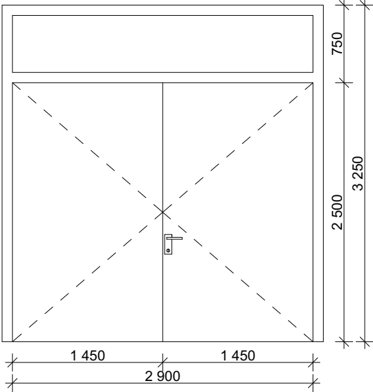
SCHÉMA Č. 4
