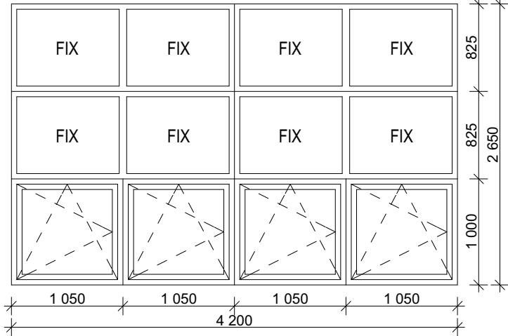
SCHÉMA Č. 3
