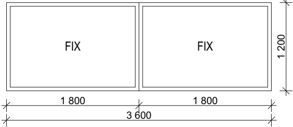
SCHÉMA Č. 4
