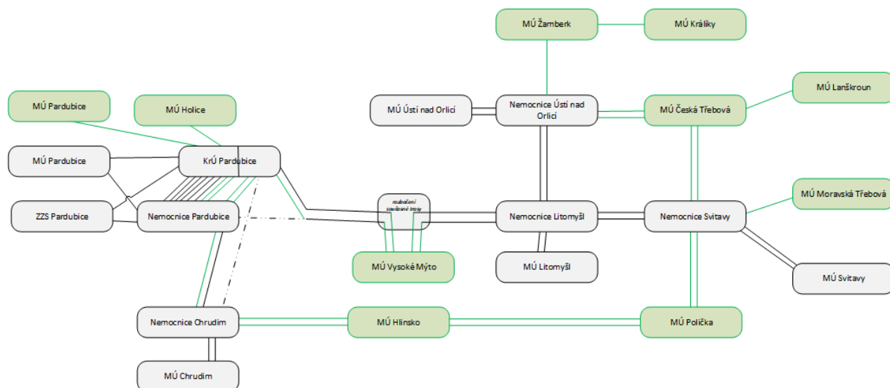
Obrázek: Předpokládaná topologie FO tras RDS 2.0
