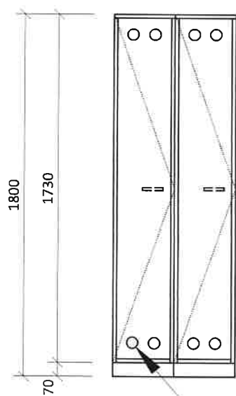
Pohled
