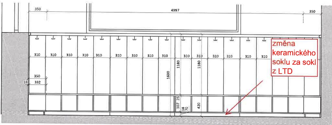
Pohled 01
