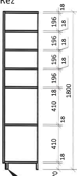
Řez
