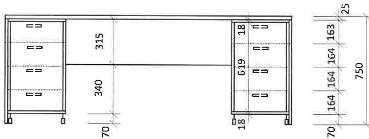
Pohled
