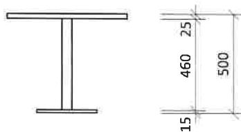
Pohled
