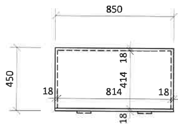
Pohled
