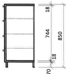
Řez
