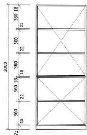
Pohled
