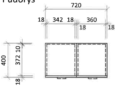
Půdorys
