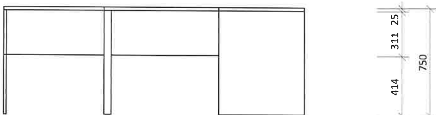
Pohled 02
