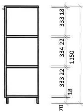
Řez
