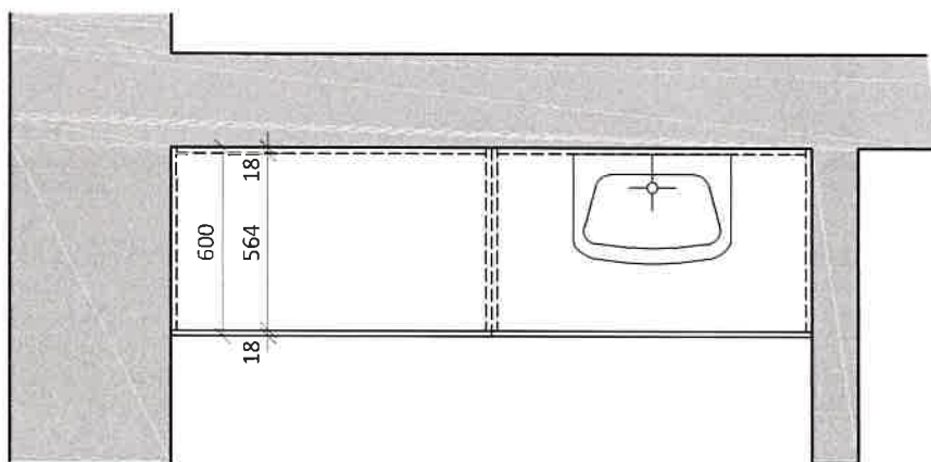
Půdorys
