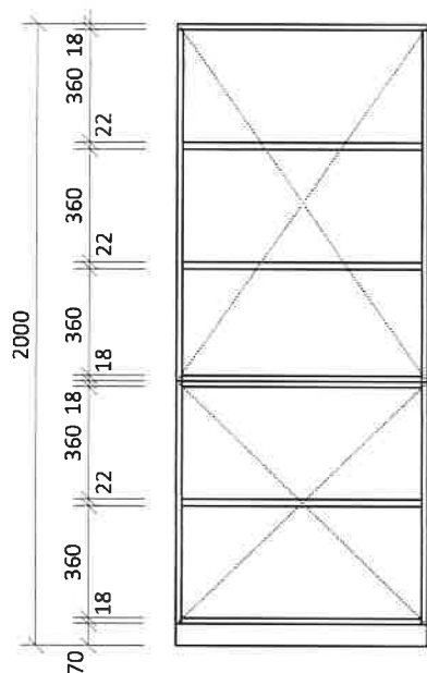
Pohled
