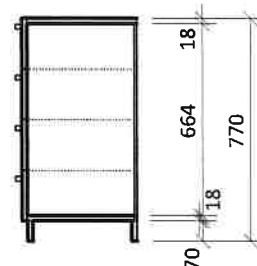
Řez
