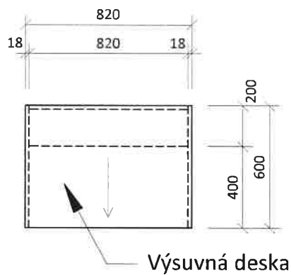
Pohled
