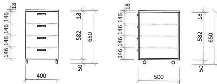
Kontejner - 1.09 C
