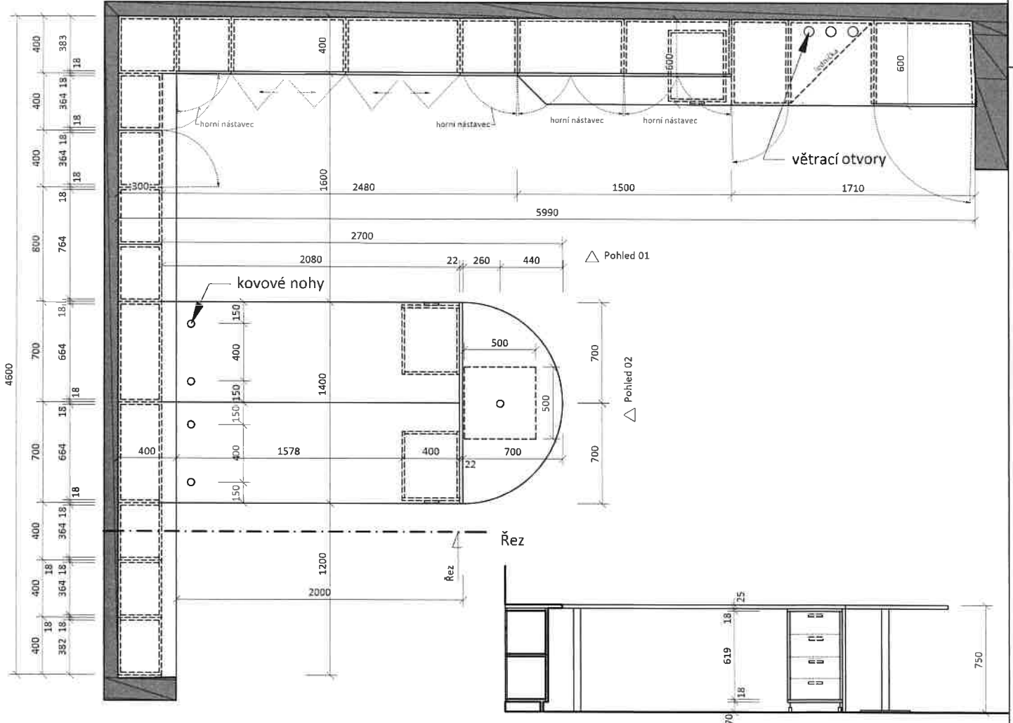
Půdorys
