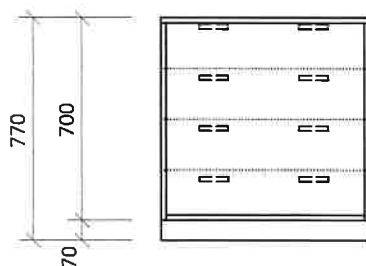
Pohled
