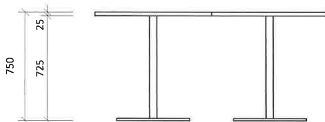
Pohled
