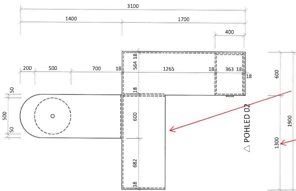
Půdorys
