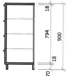
Řez
