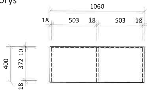
Půdorys
