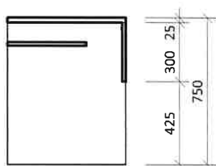
Řez
