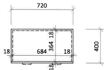
Řez
