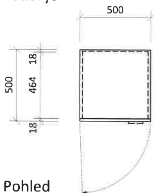
Půdorys
