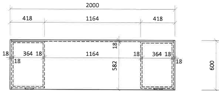
△ Pohled
