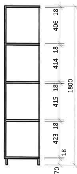
Řez
