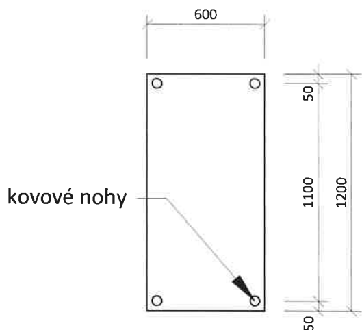
Půdorys
