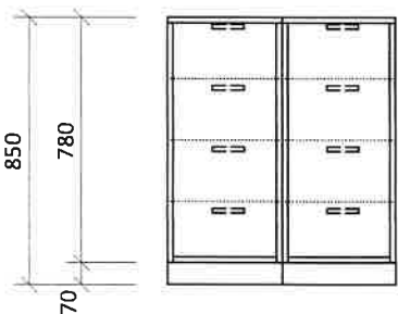
Pohled
