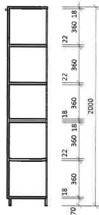
Řez
