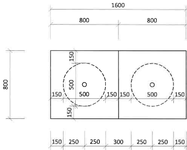
Pohled
