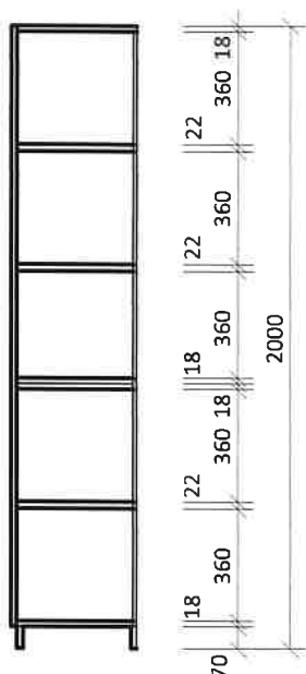
Řez
