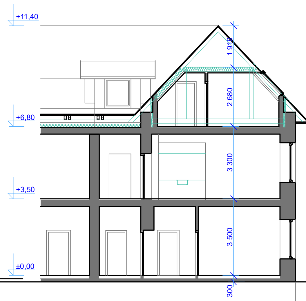
řez B/1
