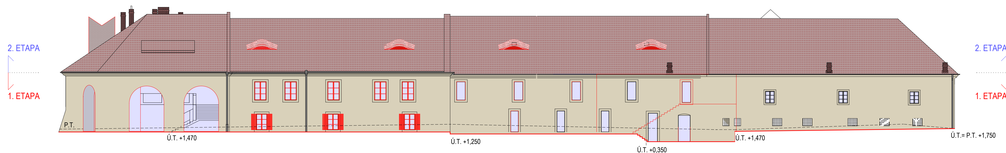
pohled severní
