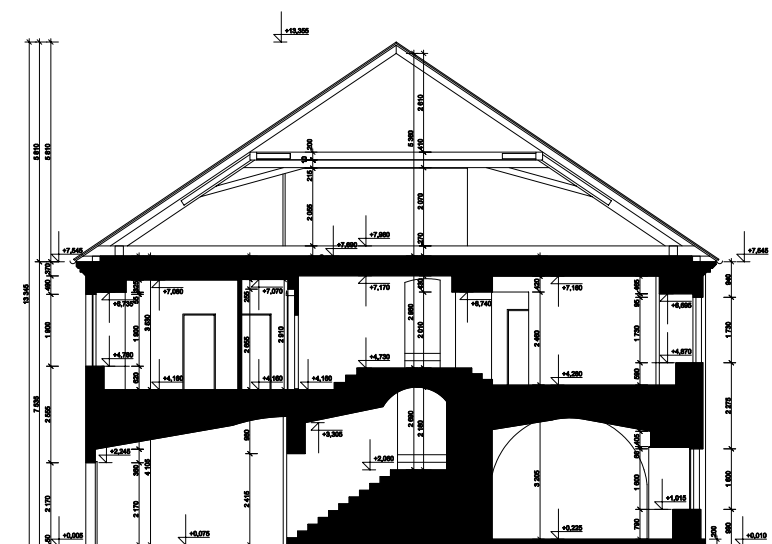
řez - stav
