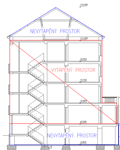
Obr. 2 Rozdělení objektu na zóny a nevytápěné prostory
